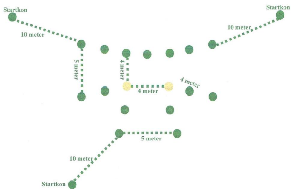
Fig 2. T-vägs korsning i klass II
